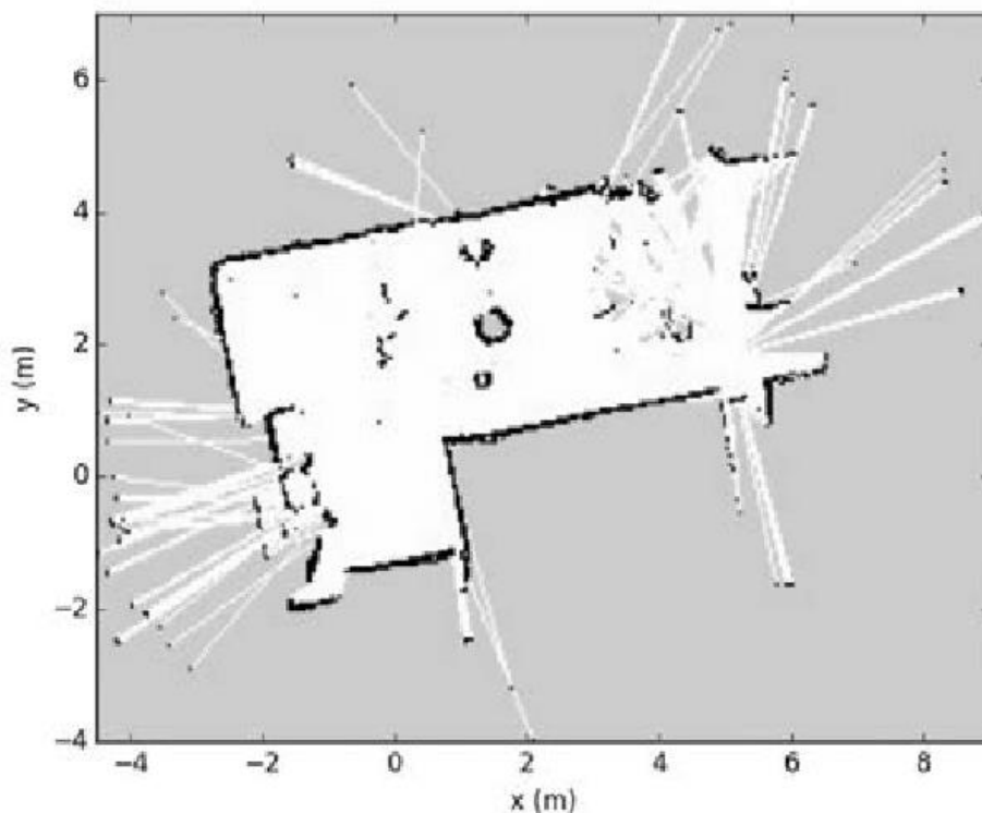
Рис. 8. GMapping
