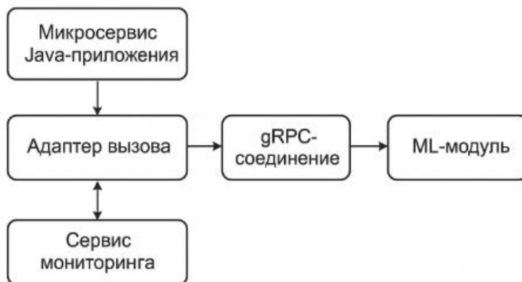
Рис. 1. Архитектура приложения
