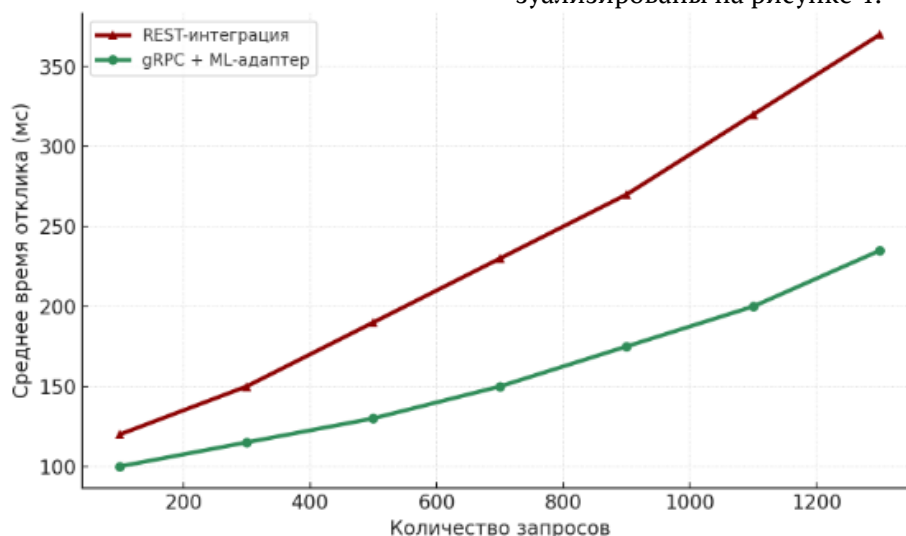
Рис. 4. Влияние модифицированной архитектуры на производительность
