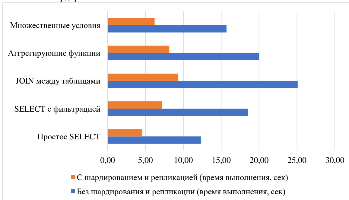
Рис. 2. Влияние шардирования и репликации на производительность запросов
