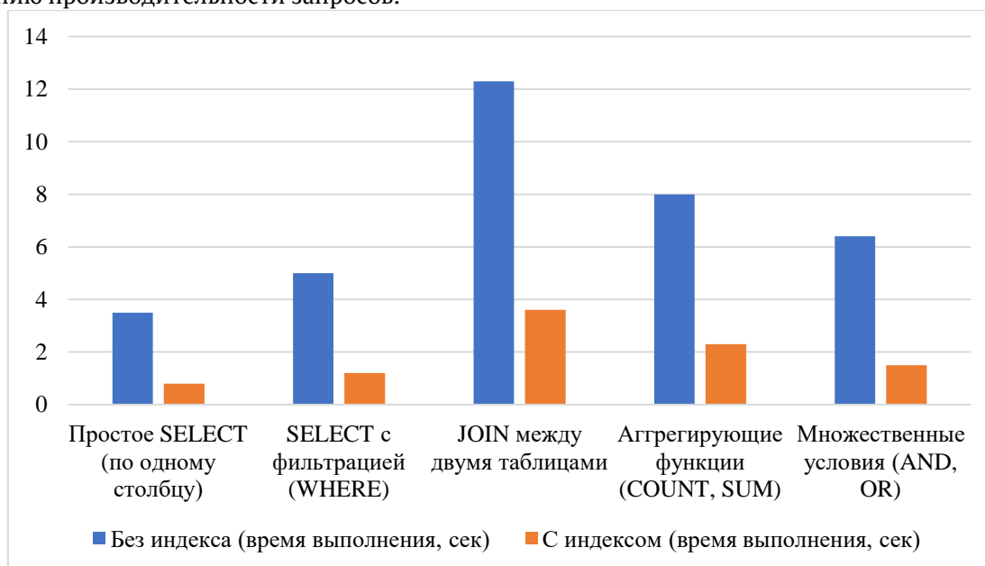
Рис. 1. Влияние индексов на производительность запросов
