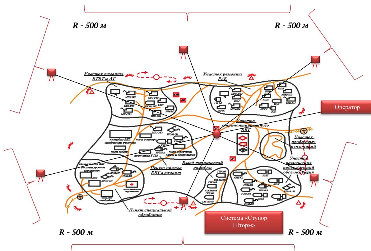
Рис. Схема охраны сборного пункта поврежденных машин
