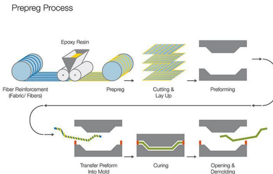
Рис. 2. Основные этапы производства препрегов
