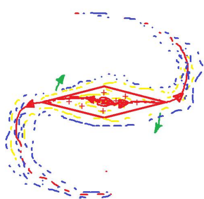
Рис. 4. А - Схема движения вещества. Б - NGC 1300 (ESO 547-31, MCG -3-9-18, UGCA 66, IRAS03174-1935, PGC 12412) – спиральная галактика с перемычкой, находится на расстоянии около 60 миллионов световых лет в созвездии Эридан
