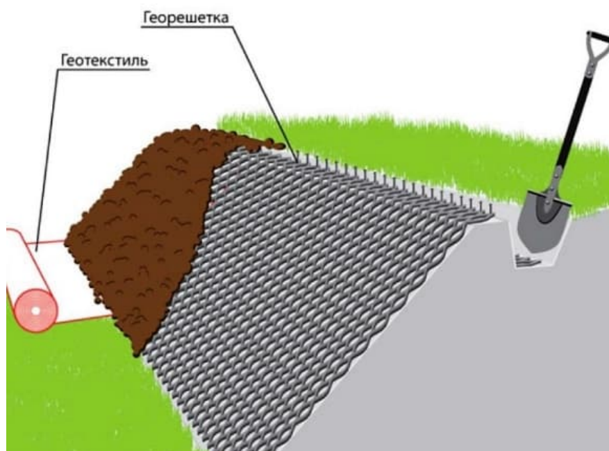
Рис. 1. Укрепление проблемных участков с помощью геосинтетических материалов
