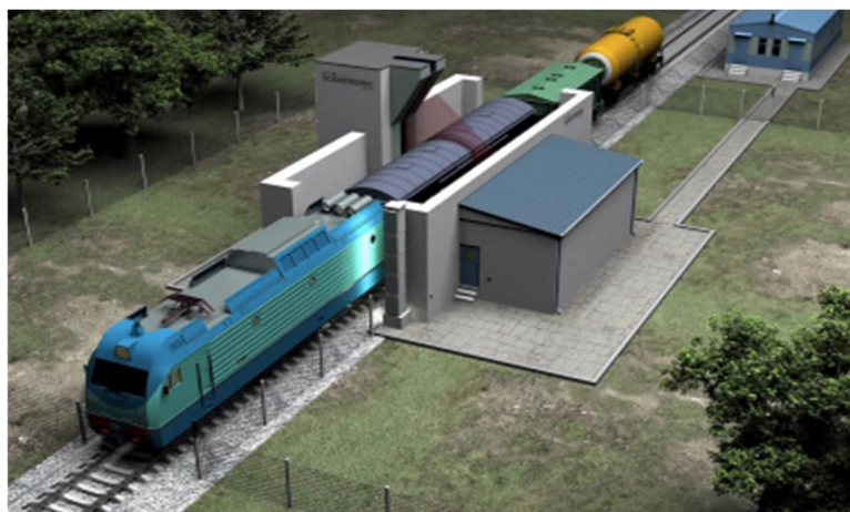
Рис. 1. Инспекционно-досмотровый комплекс для контроля железнодорожных вагонов СТ2630Т
