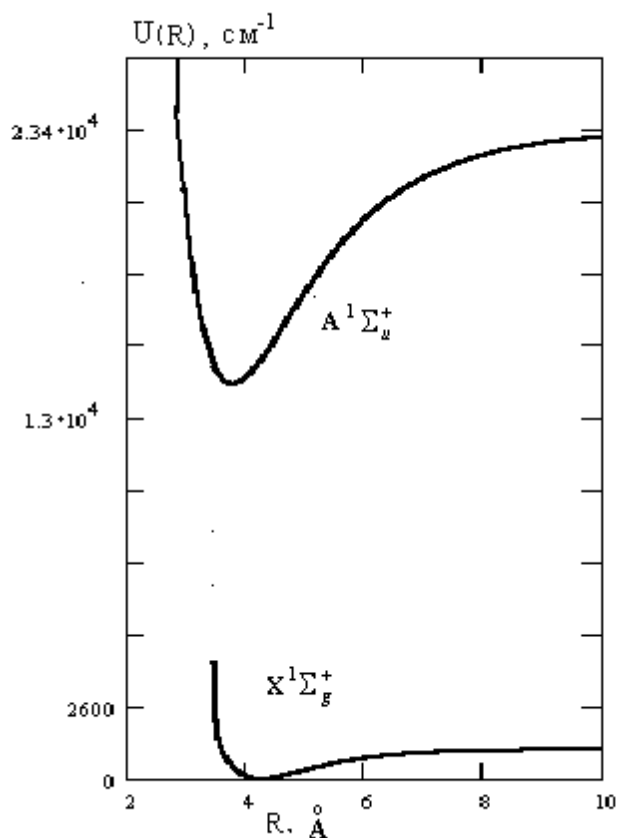
Рис. Потенциальные кривые ВОМ основного и возбужденного состояний электронного перехода A^1\Sigma_u^+ - X^1\Sigma_g^+ молекулы \text{Ca}_2
