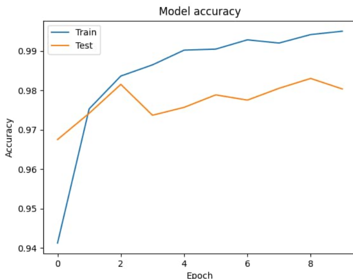
Рис. 1. График точности обучения персептрона
