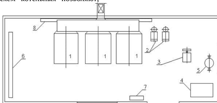
Рис. 1. Исследуемая котельная
