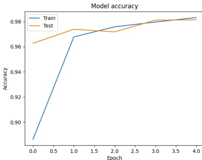
Рис. 3. График точности обучения РНС
