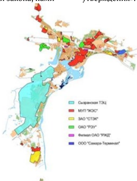
Рис. 1. Схема теплоснабжения потребителей теплоснабжающими организациями
