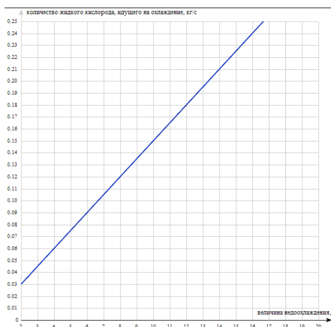
Рис. 1. Зависимость необходимого количества жидкого кислорода для впрыска от величины недоохлаждения
