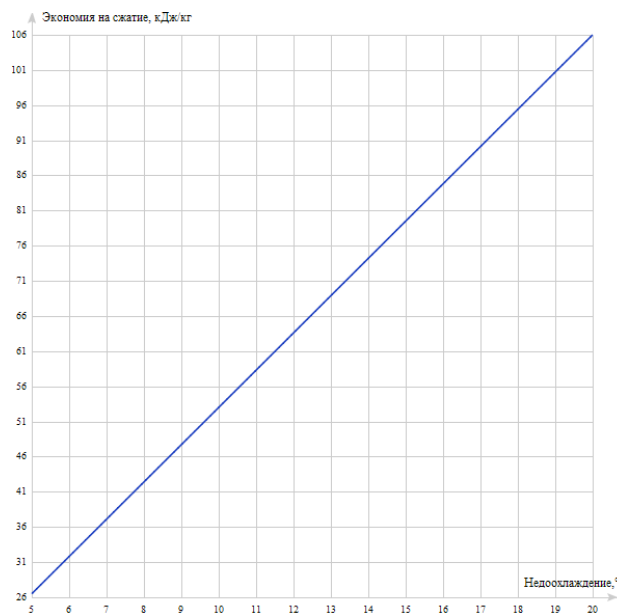
Рис. 2. Зависимость экономии энергии на сжатие при впрыске жидкого кислорода, кДж/кг жидкого кислорода
