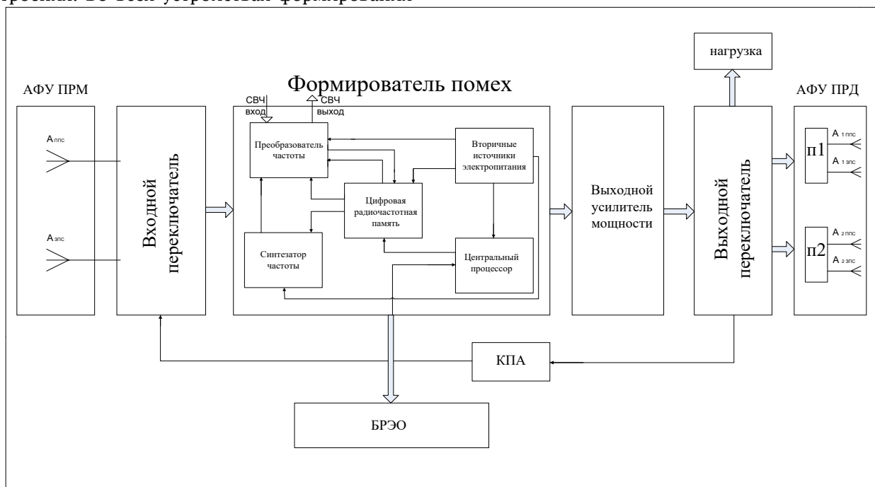
Рис. Общая структурная схема УФАП
