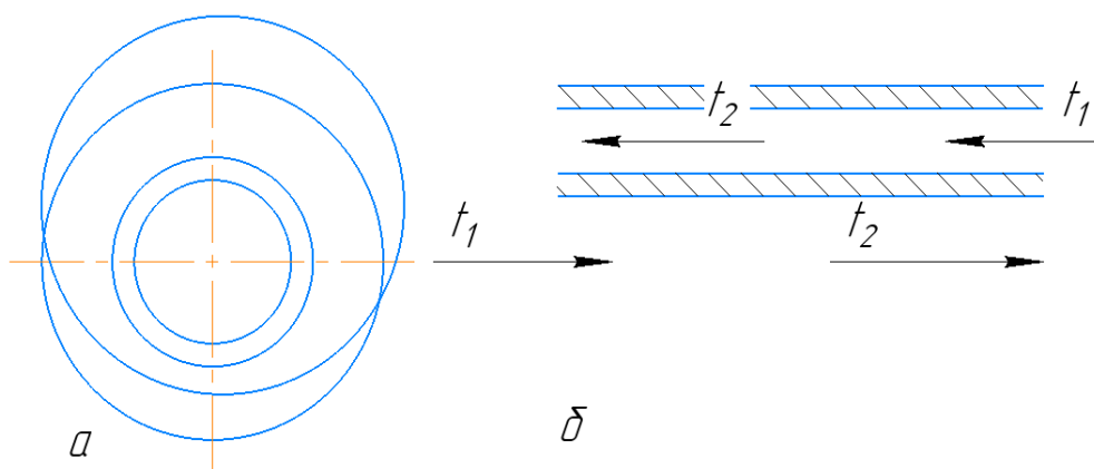
Рис. Схема тепловой сети типа труба в трубе:
