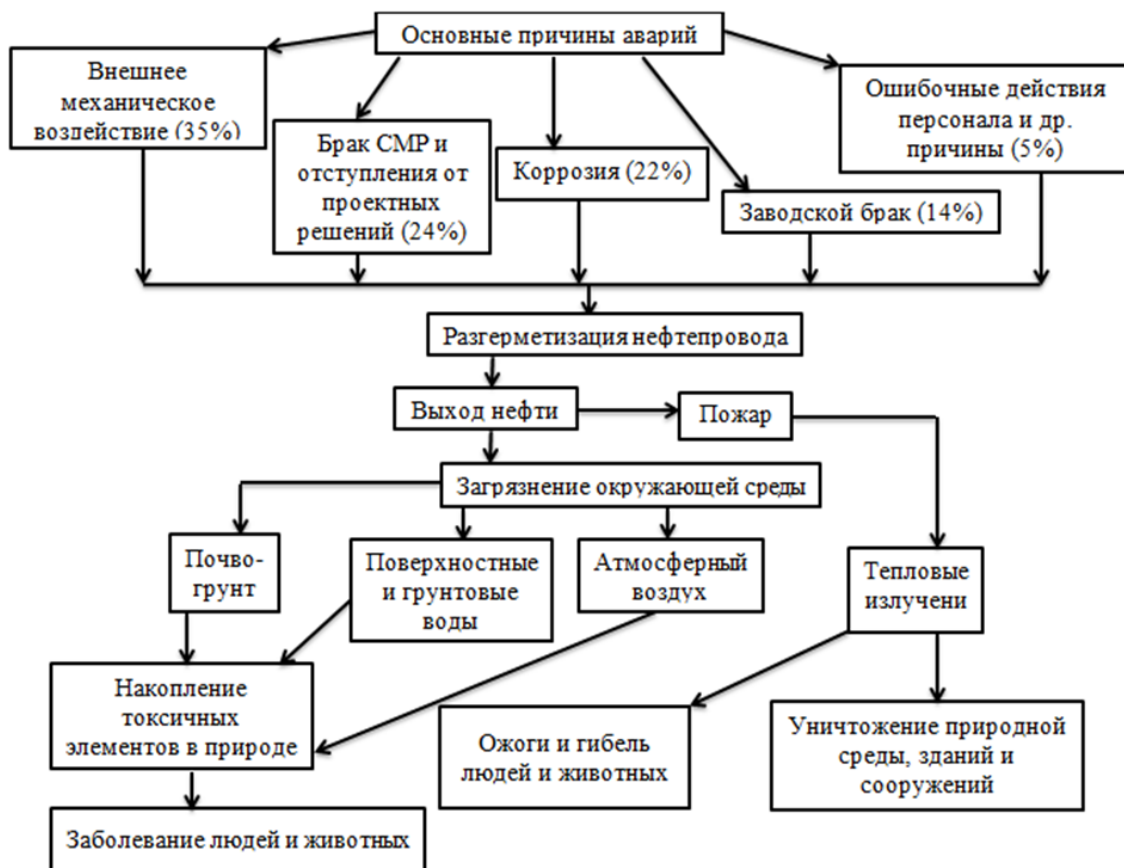
Рис. Дерево событий
