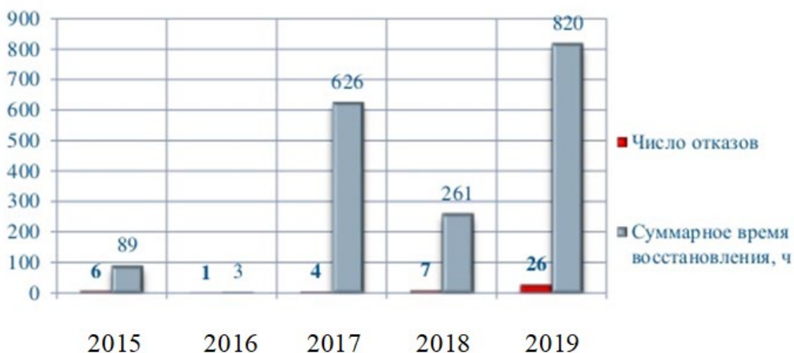
Рис. 4. Диаграмма отказов и суммарного времени восстановления за 2015-2019 гг.
