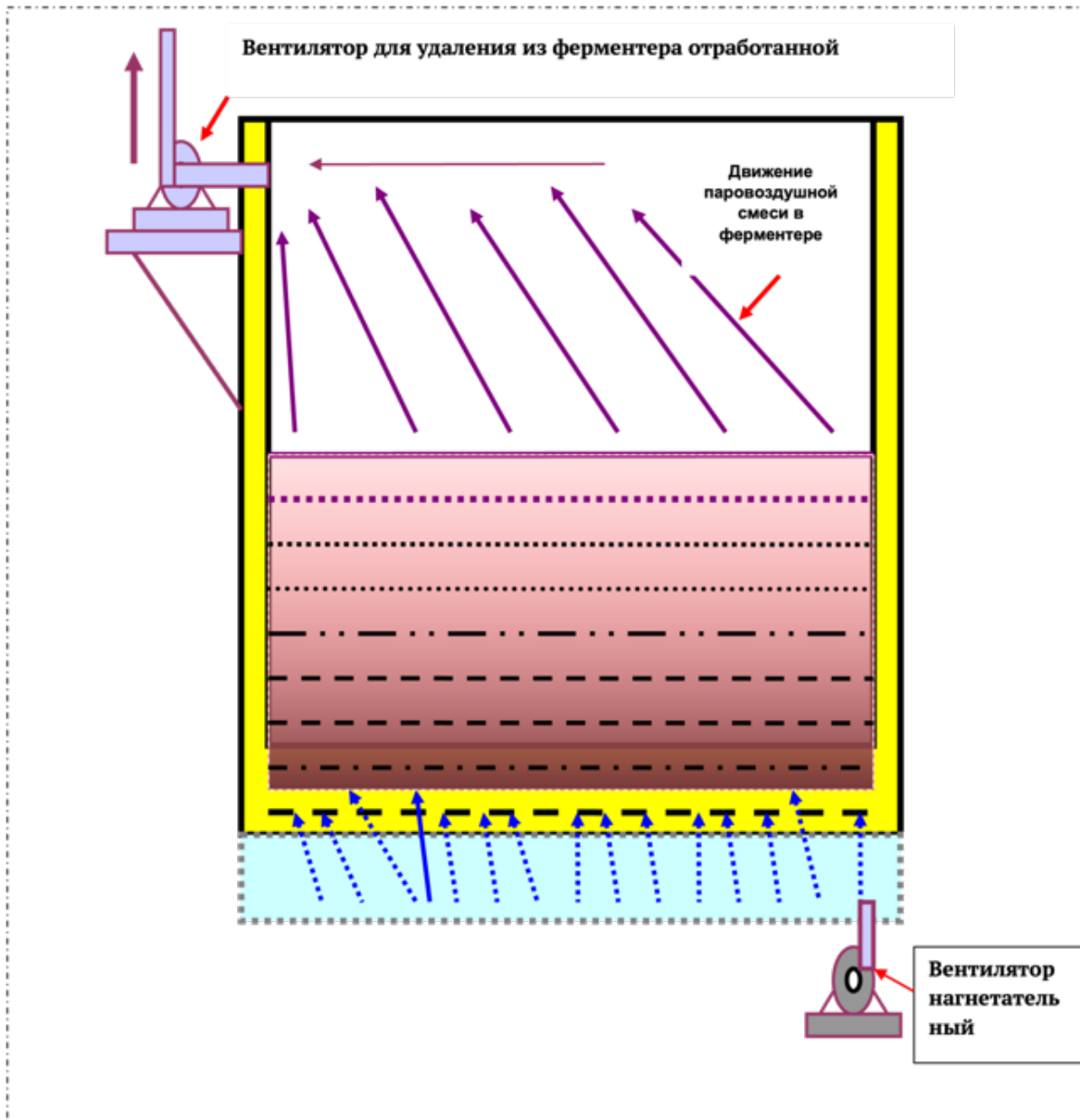
Рис. 9. Схема аэрации органической смеси в ферментере
