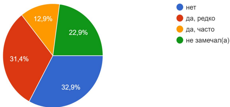
Рис. 2. Наличие чувства тревоги у опрошенных до заболевания COVID-19
