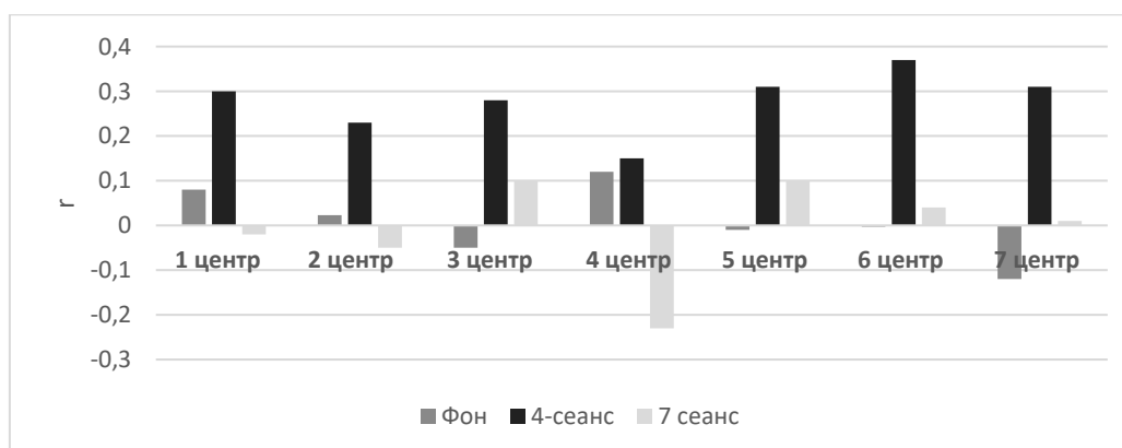
Рис. 4. Динамика корреляционной зависимости ( r ) активности энергоцентров организма волонтеров (n=24) от интенсивности потоков солнечных протонов с энергией 5 мэВ в течение 7 сеансов пребывания в «зеркальных концентраторах «энергии-времени» (Примечание: энергоцентры (чакры) 1 – Муладхара, 2 – Свадхистана, 3 – Манипура, 4 – Анахата, 5 – Вишуддха, 6 – Аджна, 7 – Сахасрара /Иванчук, Шимчишина, Трофимов, 2019/)
