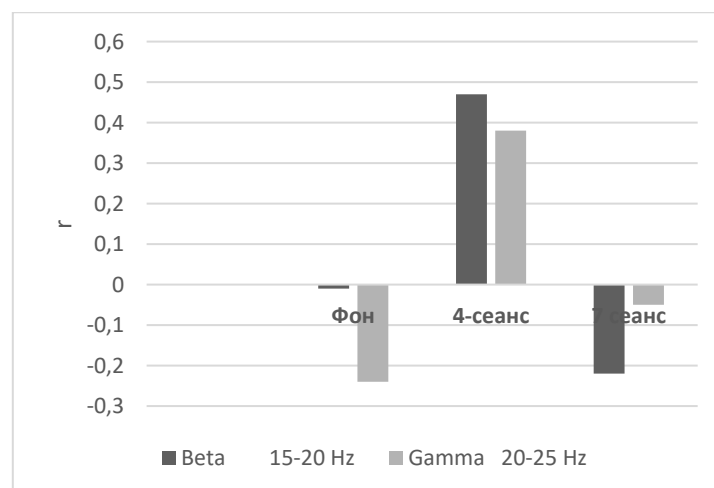
Рис. 3. Динамика корреляционной зависимости Бета – и Гамма ритмов головного мозга волонтеров ( n=24 ) от интенсивности потока протонов 5 мэВ на различных этапах зеркального тестирования /Иванчук, Шимчишина, Трофимов, 2019/
