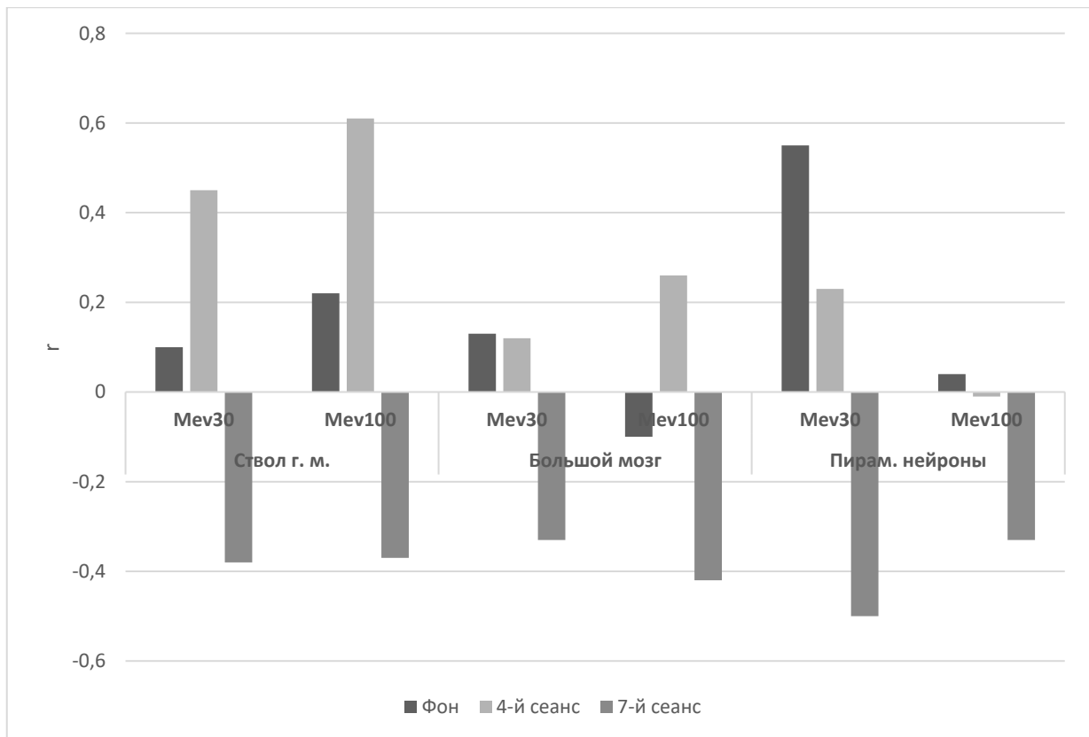
Рис. 2. Динамика корреляционной зависимости ( r ) резонансного ответа различных структур головного мозга волонтеров (по данным ДИАНЕЛ-диагностики) от интенсивности потока солнечных нейтронов (30 мэВ) и галактических протонов с энергией (100 мэВ) на различных этапах «зеркального экранирования» /Иванчук, Шимчишина, Трофимов, 2019/
