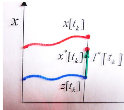
Рис. 3. Экстремальный сдвиг
