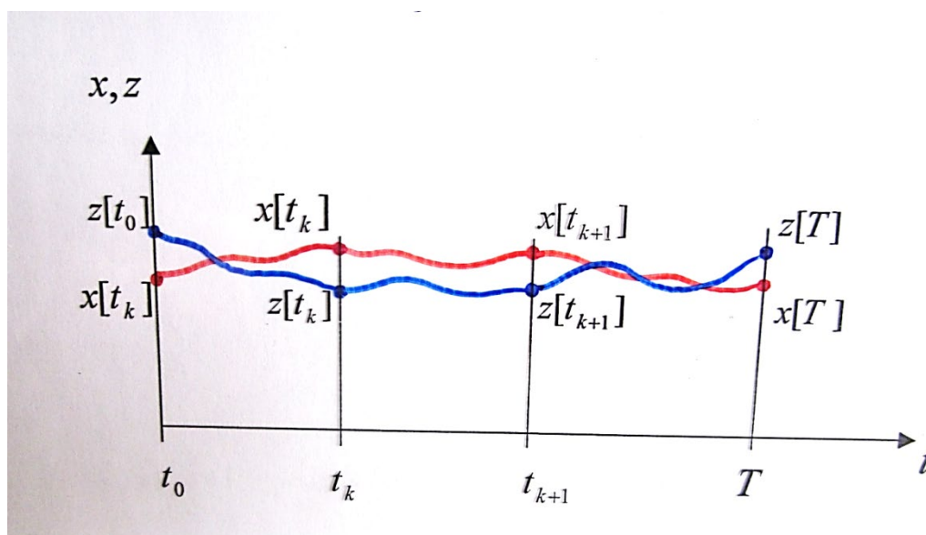
Рис. 4. Близость движений
