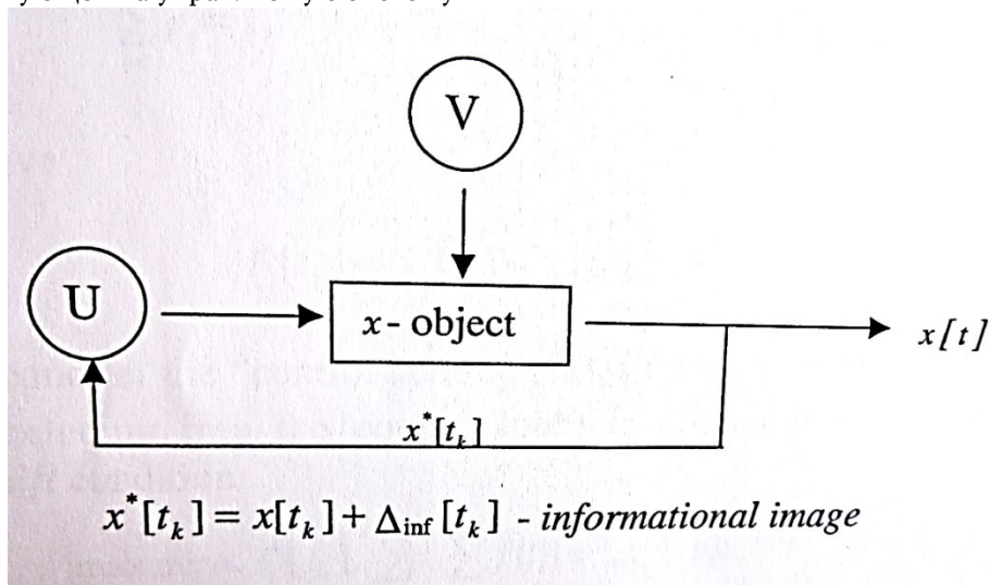
Рис. 1. Обратная связь
