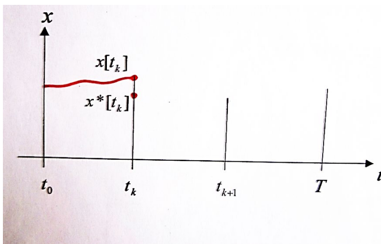
Рис. 2. Информационная ошибка
