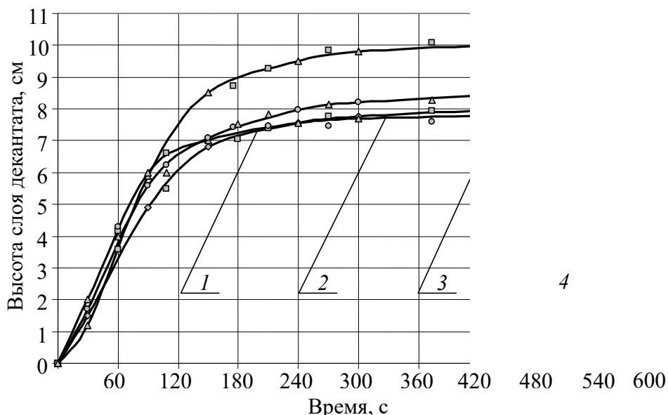
Рис. 7. Кинетические зависимости процесса разделения суспензии пигмента оранжевого Ж при использовании в качестве растворителя талой артезианской воды: 1 – без нанометаллов; 2 – с нано-Ni; 3 – с нано-Cu; 4 – с нано-Fe
