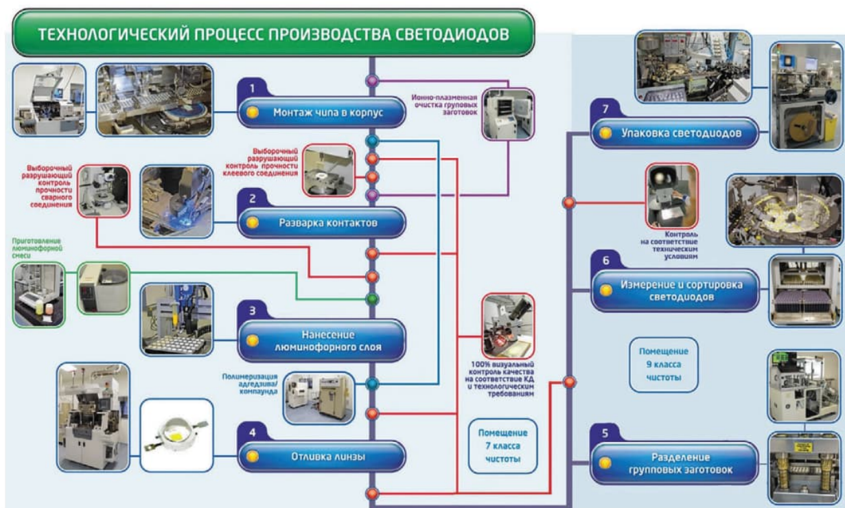
Рис. Технологический процесс производства светодиодов
