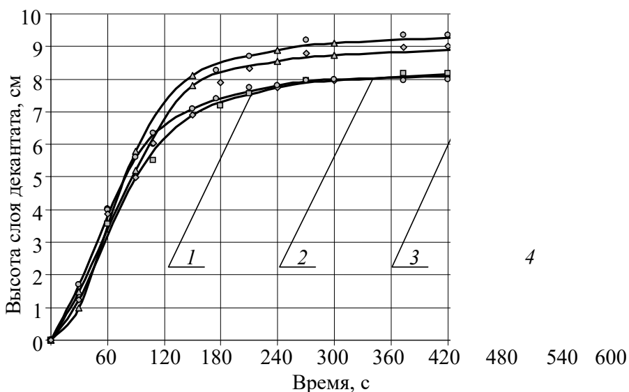
Рис. 6. Кинетические зависимости процесса разделения суспензии пигмента оранжевого Ж при использовании в качестве растворителя артезианской воды пропущенной через УСВР: 1 – без нанометаллов; 2 – с нано–Ni; 3 – с нано–Cu; 4 – с нано–Fe
