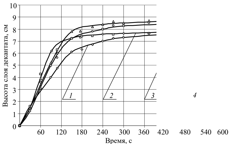
Рис. 5. Кинетические зависимости процесса разделения суспензии пигмента оранжевого Ж при использовании в качестве растворителя артезианской воды: 1 – с нано–Cu; 2 – без нанометаллов; 3 – с нано–Ni; 4 – с нано–Fe
