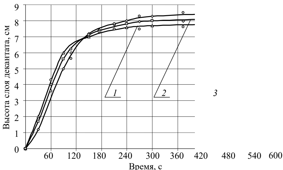
Рис. 3. Кинетические зависимости процесса разделения суспензии пигмента оранжевого Ж при введении в растворитель нанометала Ni: 1 – артезианская вода; 2 – талая артезианская вода; 3 – артезианская вода, пропущенная через УСВР
