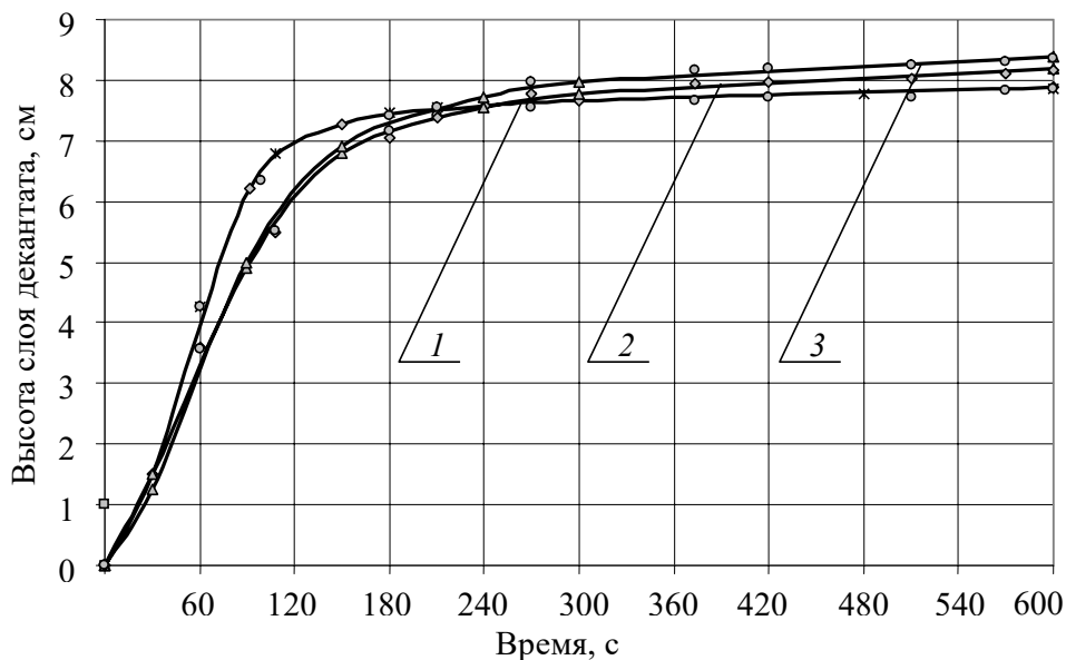
Рис. 1. Кинетические зависимости процесса разделения суспензии пигмента оранжевого Ж дисперсионная среда: 1 –артезианская вода; 2 – талая артезианская вода; 3 – артезианская вода, пропущенная через УСВР
