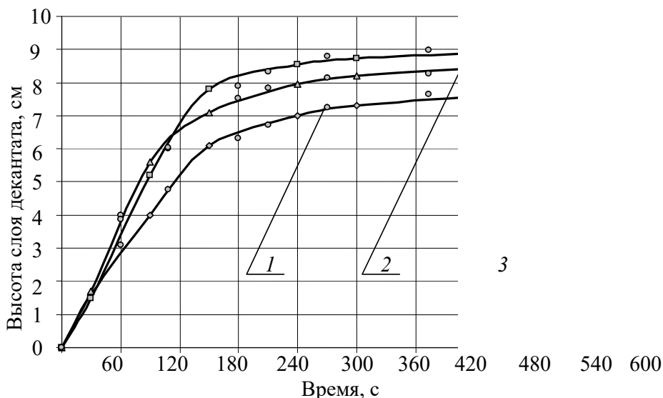
Рис. 4. Кинетические зависимости процесса разделения суспензии пигмента оранжевого Ж при введении в растворитель нанометала Cu: 1 – артезианская вода; 2 – талая артезианская вода; 3 – артезианская вода, пропущенная через УСВР
