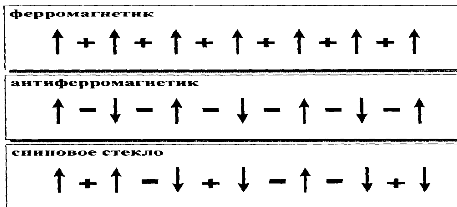
Рис. 1. Знаки связей между спинами в ферромагнетике, антиферромагнетике и спиновом стекле
